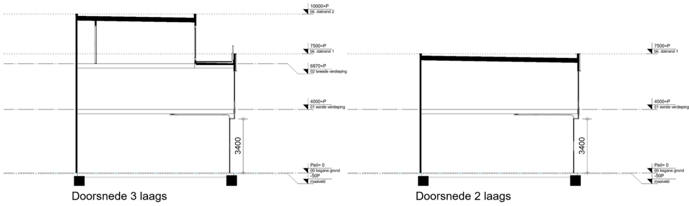
Doorsnede 3 laags
