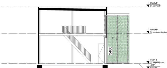
Doorsnede 2 laags
