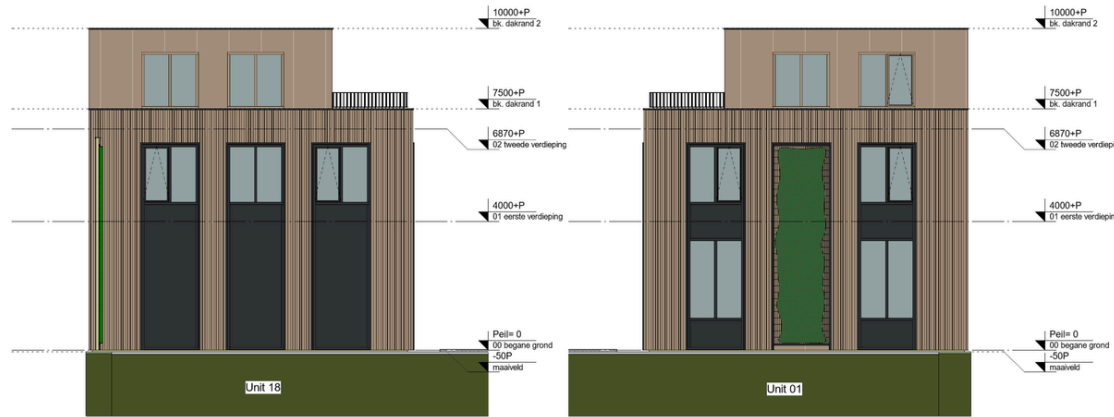
Linkergevel blok A
