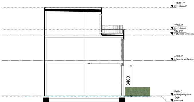
Doorsnede 3 laags
